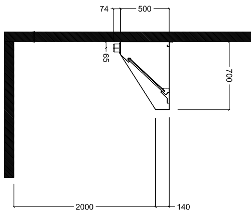
Zij aanzicht
